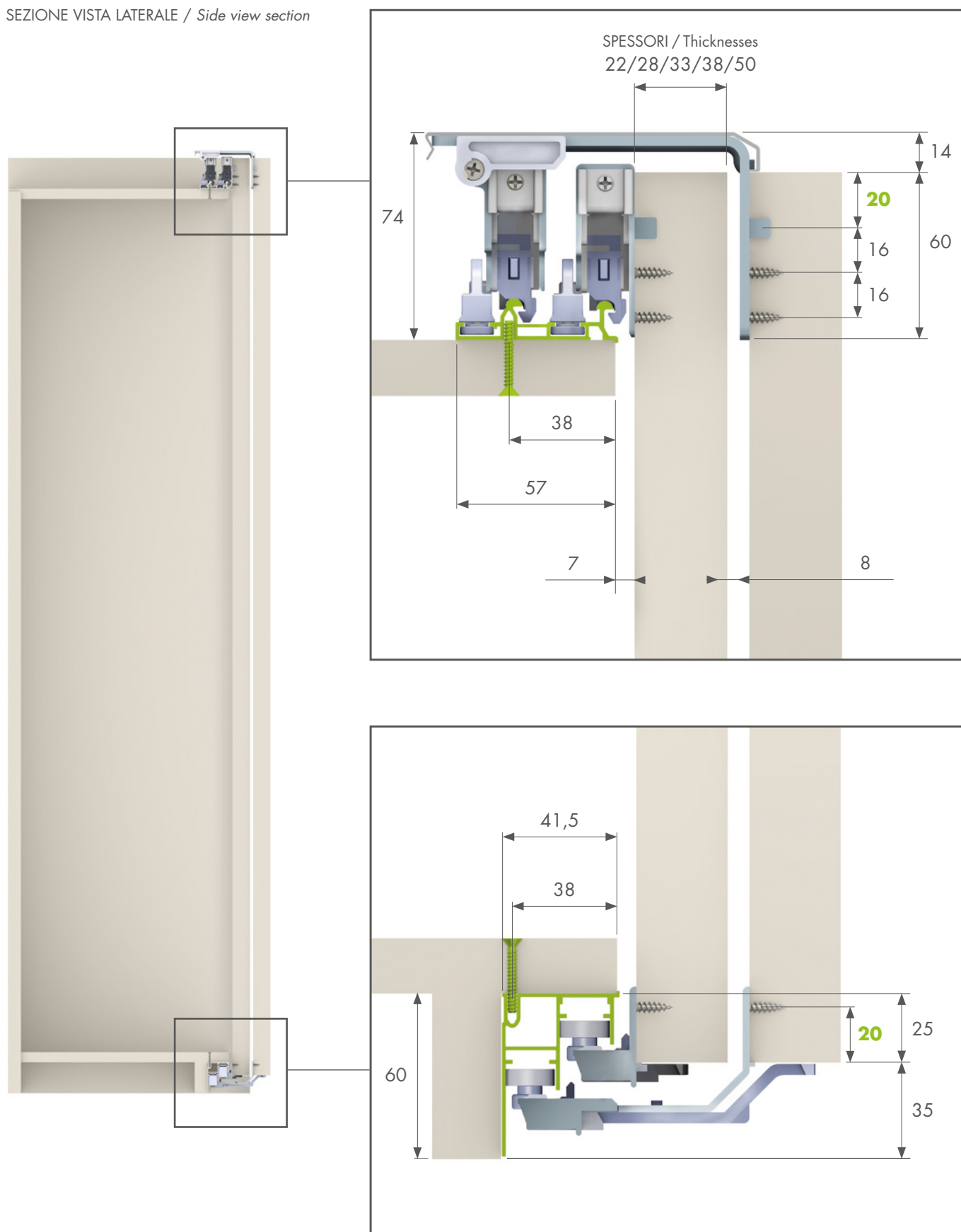
SEZIONE VISTA LATERALE / Side view section
